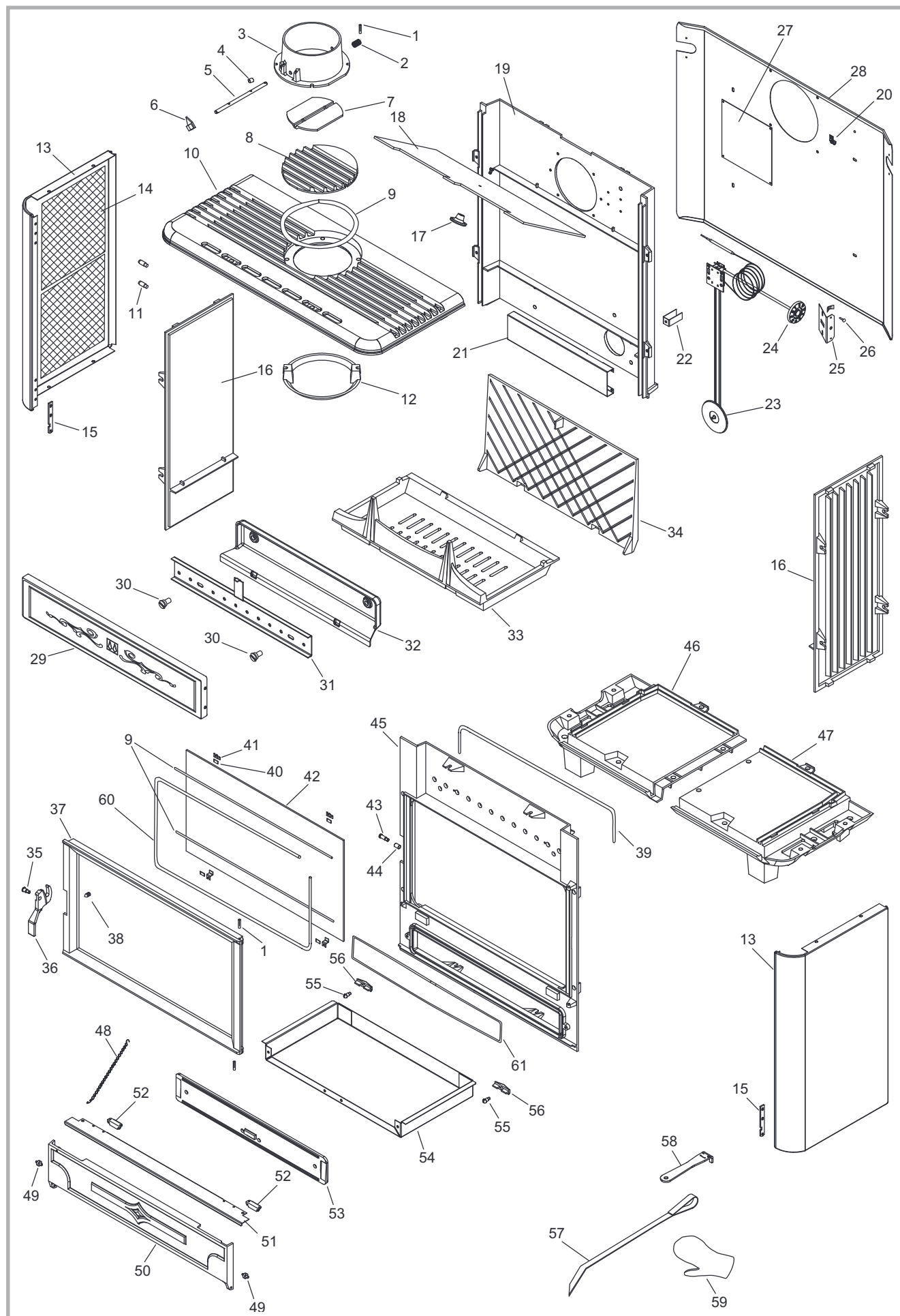
Figure 9 - Vue éclatée
