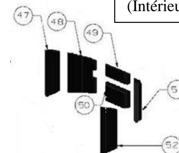
Version 8 KW (Intérieur fonte)
