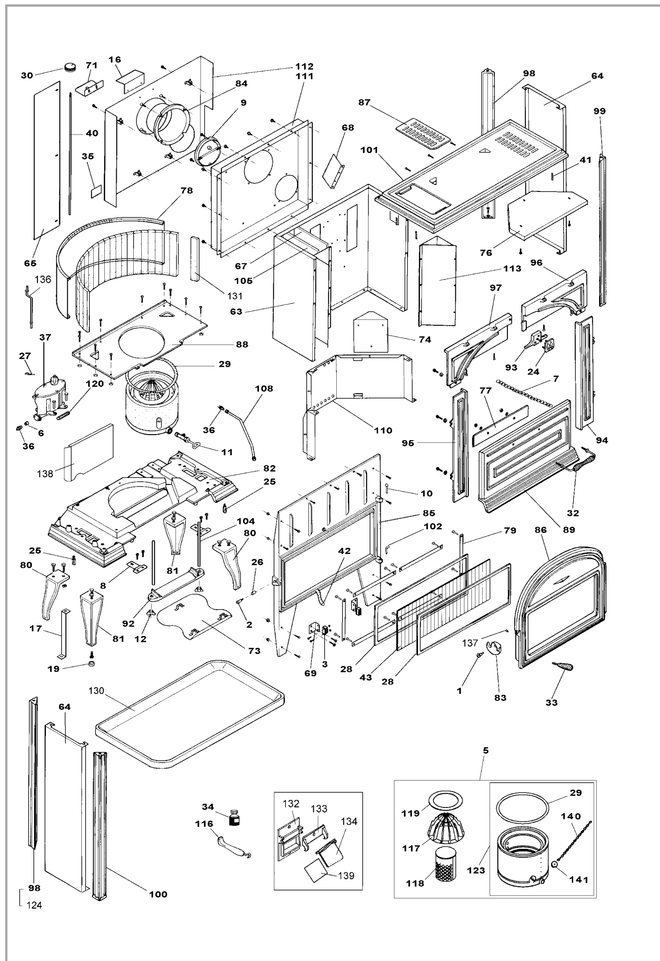
Fig. 14 - Vue éclatée de l'appareil
