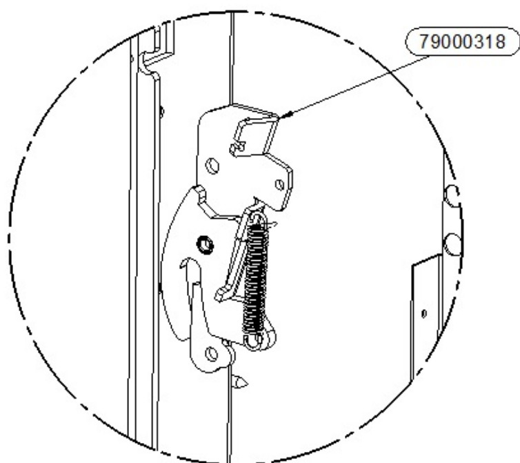
DETTAGLIO A
