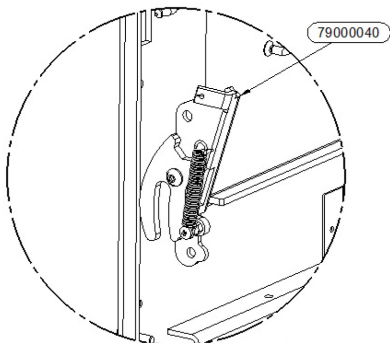
DETTAGLIO D
